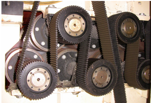
15 ROLL WEB DRAFTER
